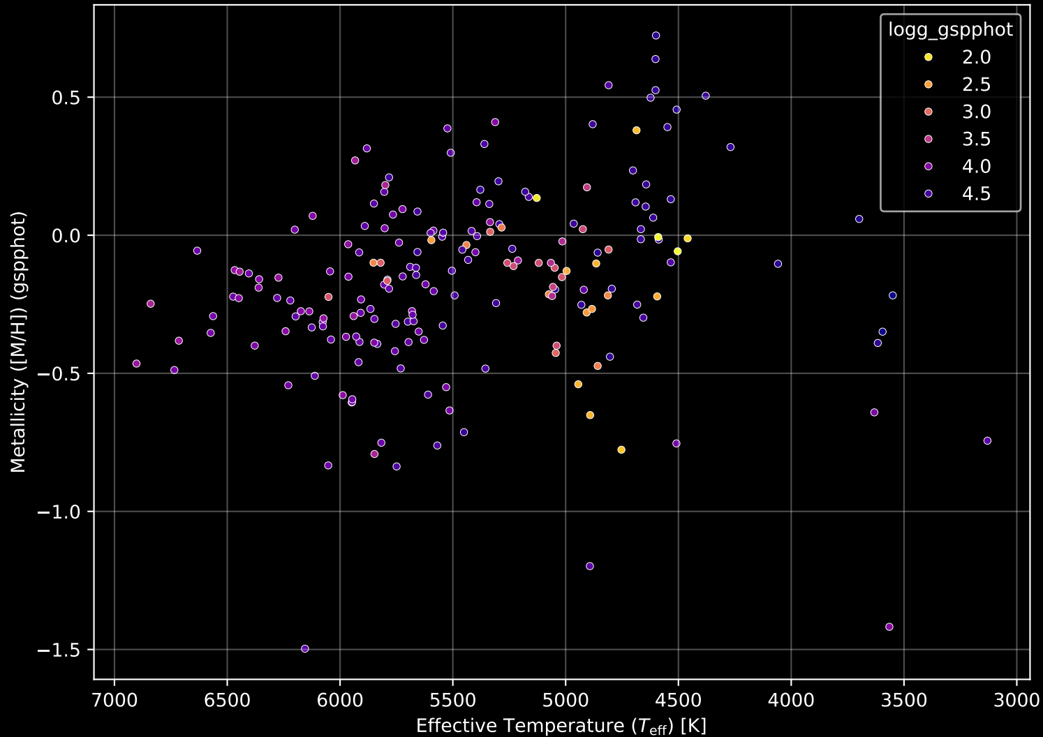
APOGEE DR17 Field: [065+48_MGA] Stellar Population Parameters (n= 197)
